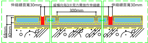
伸縮縫施作示意圖
