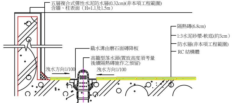
施作剖面詳圖
